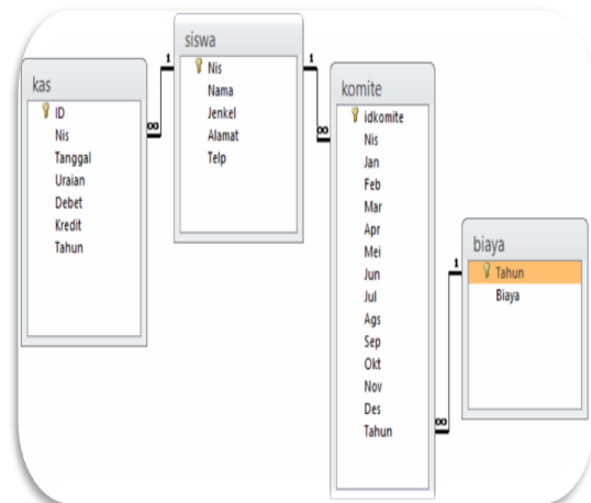
Gambar 6. Relasi Tabel ERD
