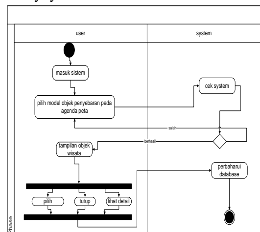
Gambar 6. Activity diagram kelola data kategori
