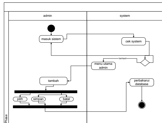
Gambar 5. Activity diagram kelola lokasi
